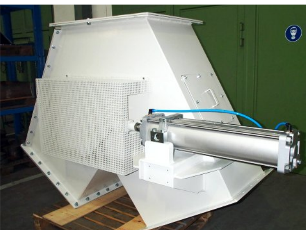
Ходовой распределитель с пневматическим приводом
