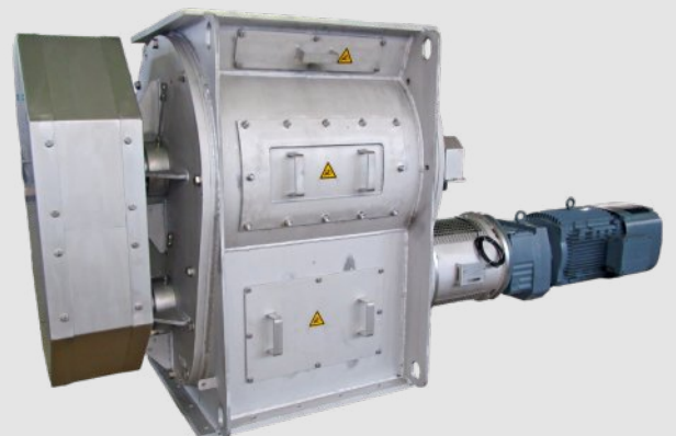
Самоочистной ячейковый питатель ZRS-R
