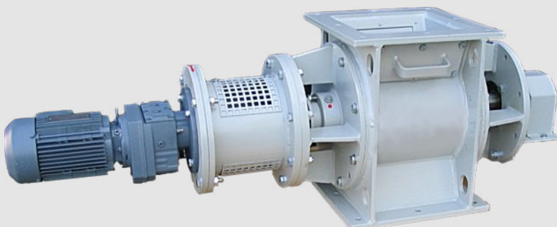
Ячейковый питатель с моторредуктором
